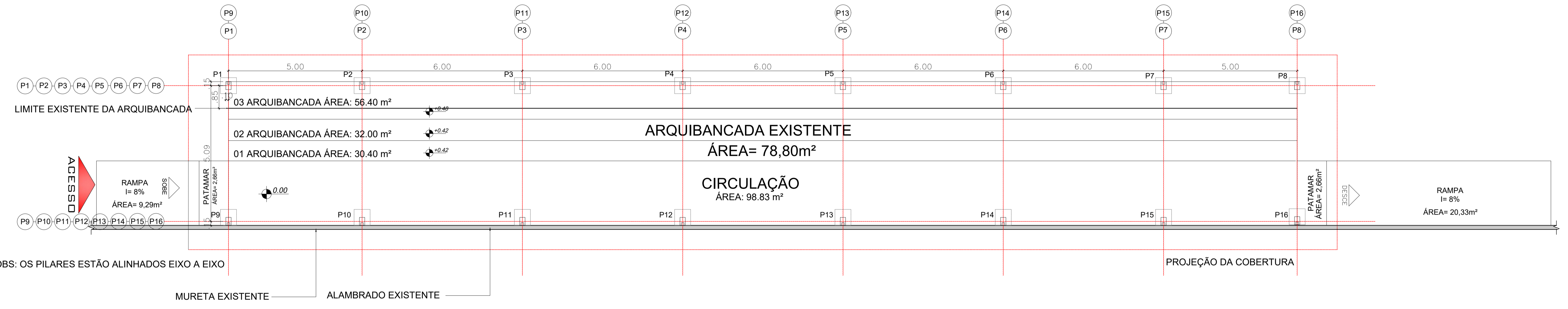
LOCAÇÃO DE SAPATAS E PILARES esc: 1/75
