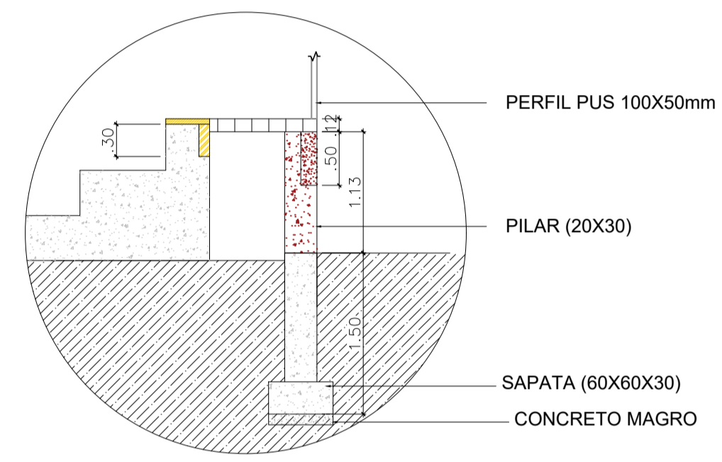
DETALHE CORTE ESTRUTURAL esc: 1/20
