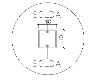
DETALHE PILAR EM PUS 50X50mm (2X) esc: 1/20
